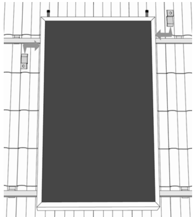
Abb. 37: Die oberen Quickies wieder lösen. Einen dieser Quickies von oben und einen von unten über die obere C-Profil-Schiene schieben und fest verschrauben.
