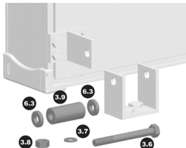
Abb. 74: Sechskantschrauben M10 (3.6/ 4.7), kleine Distanzhülsen (6.3), große Distanzhülsen (3.9/ 4.10), Federringe (3.7/ 4.8) und Sechskantmuttern M10 (3.8/ 4.9) zur Kollektorbefestigung bereitlegen.
