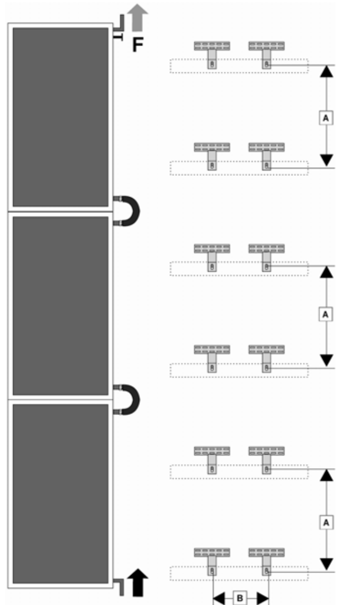
Abb. 9: Variante 3 hochkant übereinander Außenmaße Kollektorfeld: 1,16x5,61 m A 1,20-1,75 m B 0,80-1,05 m
