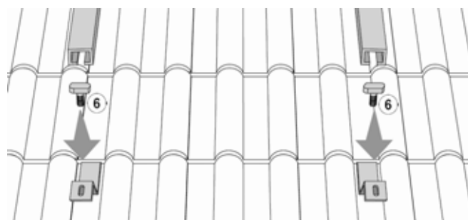
Abb. 39: Das C-Profil mit Hammerkopfschrauben ⑥ auf die Sparrenanker montieren. Achtung: Im Bereich der Sparrenanker können die Quikies zur Kollektorbefestigung nicht in die Schiene einrasten. Deshalb die Sparrenanker nie mittig zwischen zwei Kollektoren montieren.
