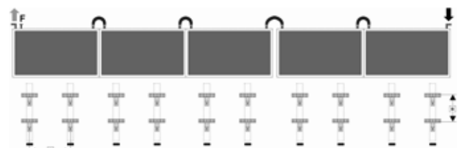
Abb. 16: Variante 2 quer nebeneinander Außenmaße Kollektorfeld: 9,35x1,16 m A 1,20-1,75 m B 0,80-1,05 m
