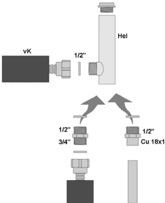
Abb. 54: Das T-Stück mit Entlüfter wird an dem Flexrohr unter dem Dach montiert. Der Übergang vom T-Stück zur weiteren Verrohrung erfolgt über einen Löt nipple (für Cu-Rohr) bzw. einen Reduziernippel (bei Einsatz von Flexrohr).
