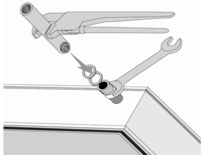
Abb. 55: Bei der Montage des Entlüfters auf dem Dach muss zunächst das T-Stück mit vormontiertem Entlüfter auf den Kollektorfeldanschlüssen befestigt werden (sowohl im Vor- als auch im Rücklauf). Zwischen Kollektor und T-Stück muss eine Dichtung eingelegt werden. Zur optimalen Ausrichtung des Anschlusses kann eine zweite Dichtung eingelegt werden.
