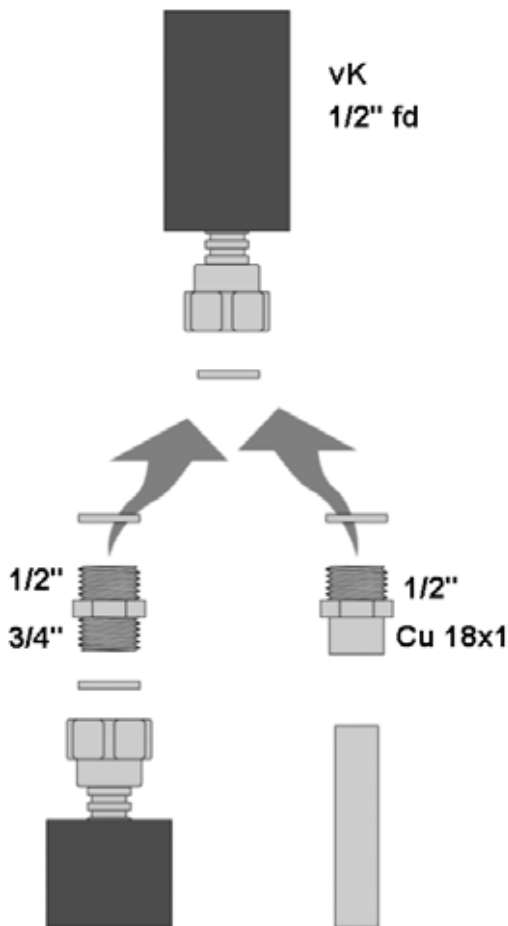
Abb. 58: Bei Übergang auf Kupferrohr wird der Löt nipple eingesetzt, bei Übergang auf Flexrohr kommt der Reduziernippel zum Einsatz. Dichtringe nicht vergessen!
