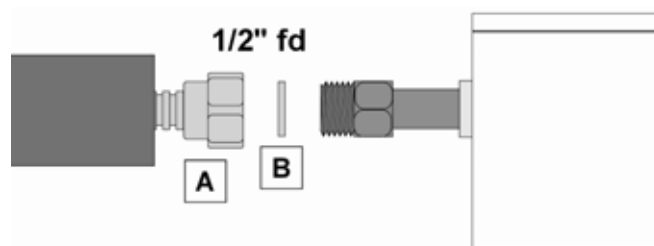
Abb. 53: Beim Anschluss der Edelstahlwellrohre Ⓐ auf den korrekten Sitz der Flachdichtung Ⓑ achten.
