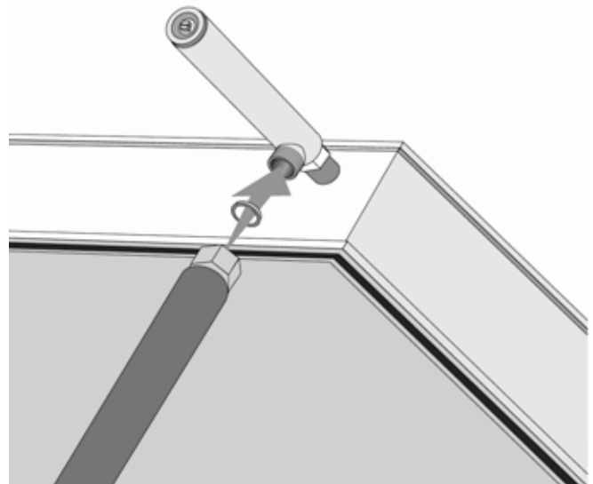
Abb. 56: Anschließend wird das lange Edelstahlwellrohr (900 mm) mit dem T-Stück verbunden.
