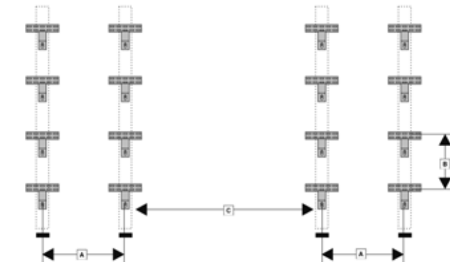
Abb. 17: Variante 1 quer 2-spaltig Außenmaße Kollektorfeld: 3,94x3,48 m A 1,20-1,75 m B 0,80-1,05 m C 1 Dachsparrenabstand
