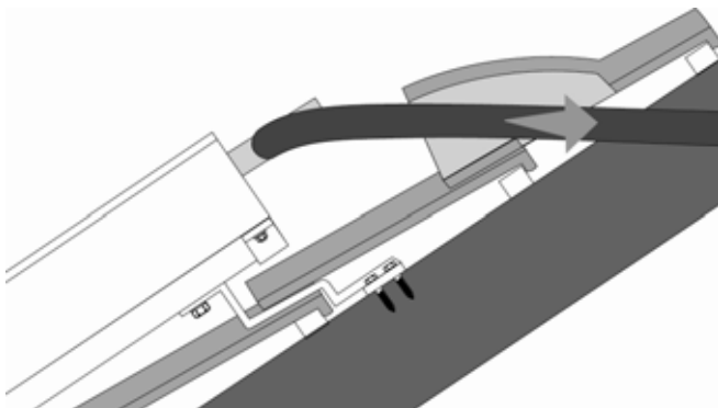
Abb. 57: Das Edelstahlwellrohr wird dann durch den Lüftungziegel geführt. Der weitere Anschluss richtet sich nach Verrohrung mit Flexrohr oder mit Kupferrohr.
