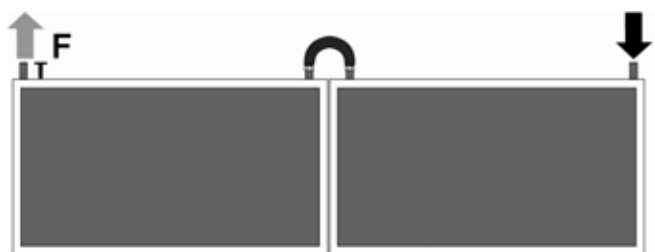
Abb. 5: Variante 3 hochkant übereinander Außenmaße Kollektorfeld: 1,16x3,74 m A 1,20-1,75 m B 0,80-1,10 m
