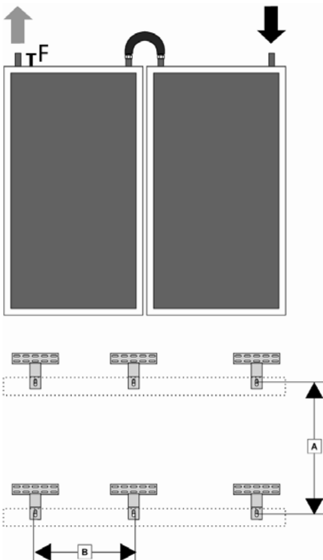
Abb. 3: Variante 1 (Standard) hochkant nebeneinander Außenmaße Kollektorfeld: 2,32x1,87 m A 1,20-1,75 m B 0,80-1,10 m
