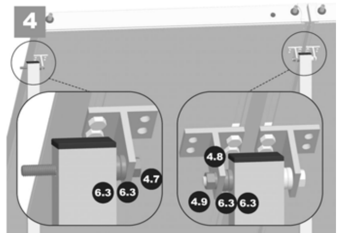
Abb. 79: Kollektor zu den Trägerrohren (2) neigen. Erst zwei kleine Distanzhülsen (6.3), dann den Kollektor mit T-Stück (6.1) und folgend Federling (4.8) und Sechskantmutter M10 (4.9) auf der vormontierten Sechskantschraube M10x100 mm (4.7) befestigen. Zweites T-Stück mittels Sechskantschraube M10x100 mm (4.7) und zwei kleiner Distanzhülsen (6.3) vormontieren. Die Sechskantschrauben M10x100 mm (4.7) zwischen den Kollektoren festziehen.
