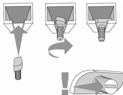
Abb. 39: Das C-Profil mit Hammerkopfschrauben ⑥ auf die Sparrenanker montieren. Achtung: Im Bereich der Sparrenanker können die Quikies zur Kollektorbefestigung nicht in die Schiene einrasten. Deshalb die Sparrenanker nie mittig zwischen zwei Kollektoren montieren.
