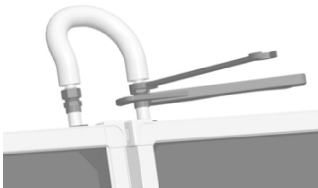
Abb. 81: Die vorher zurückgeschobenen Dämmschläuche über die Anschlüsse bis an das Kollektorgehäuse schieben.
