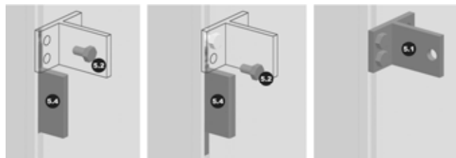
Abb. 70: Vier T-Stücke (5.1/ 6.1) je Kollektor mit Sechskantschrauben M8 (5.2/ 6.2) an den Vierkantmuttern in der Nut auf der Kollektorrückseite vormontieren. Dazu die erste Vierkantmutter mit Hilfe der langen Seite der Montagehilfe ausrichten. Das T-Stück ansetzen und eine Sechskantschraube einschrauben. Durch drehen der Montagehilfe die zweite Vierkantmutter ausrichten und eine weitere Sechskantschraube einschrauben.
