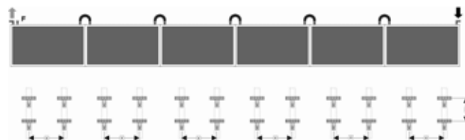
Abb. 22: Variante 6 quer 1-reihig Außenmaße Kollektorfeld: 11,22x1,16 m A 1,20-1,15 m B 0,80-1,05 m
