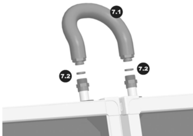
Abb. 80: Die Kollektoren (1) miteinander in Reihe verbinden. Dazu Verbindungsleitung (7.1) mit Dichtung (7.2) an entsprechende Kollektoranschlüsse montieren. Dabei auf korrekten Sitz der Dichtung achten.
