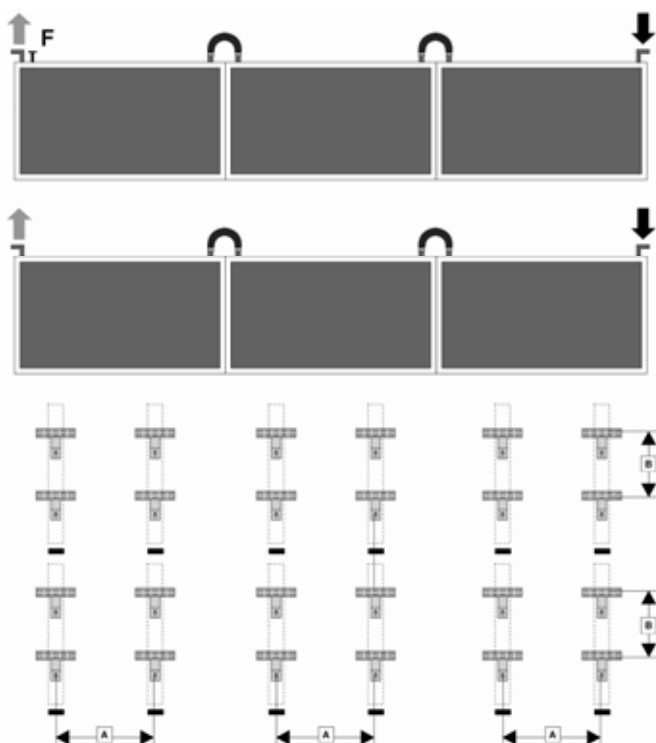
Abb. 21: Variante 5 quer 2-reihig Außenmaße Kollektorfeld: 5,61x2,52 m A 1,20-1,75 m B 0,80-1,05 m 4 Dachdurchführungen
