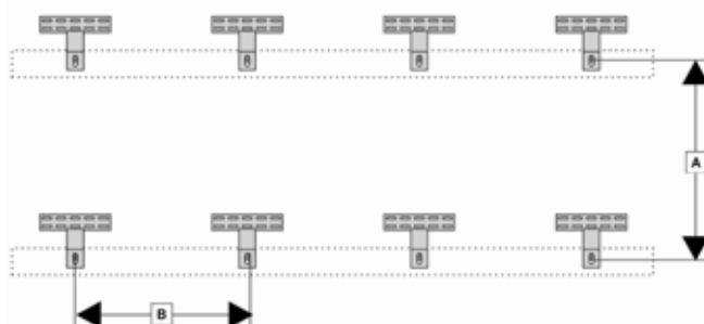
Abb. 7: Variante 1 hochkant nebeneinander Außenmaße Kollektorfeld: 3,48x1,87 m A 1,20-1,75 m B 0,80-1,10 m
