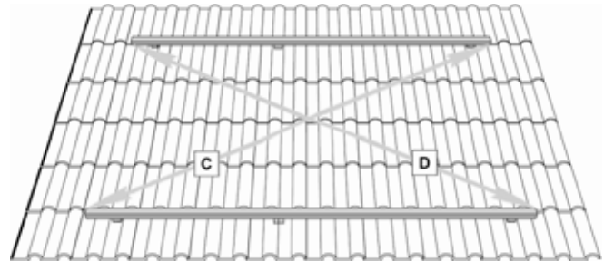
Abb. 33: Die Schienen sind parallel ausgerichtet, wenn Maß c = d (z.B. mit Schnur vermessen). Bei korrekter Ausrichtung können die Schienen fest verschraubt werden.
