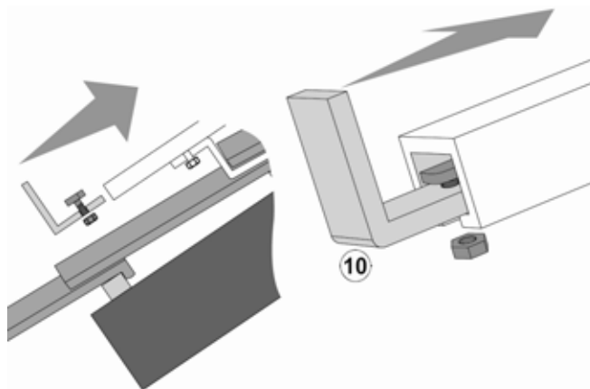
Abb. 44: Vor der Kollektormontage wird das L-Stopp-Profil ⑩ in die untere Öffnung der C-Profile gesteckt und mit Hammerkopfschrauben befestigt.
