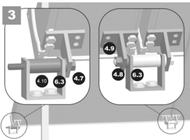
Abb. 78: Erst eine kleine Distanzhülse (6.3), dann den Kollektor mit T-Stück (6.1) und folgend Federling (4.8) und Sechskantmutter (4.9) auf der vormontierten Sechskantschraube M10x100 mm (4.7) zwischen den Kollektoren befestigen. Zweites T-Stück auf dem zweiten U-Stück mittels Sechskantschraube M10x100 mm (4.7), kleiner Distanzhülse (6.3) und großer Distanzhülse (4.10) vormontieren.
